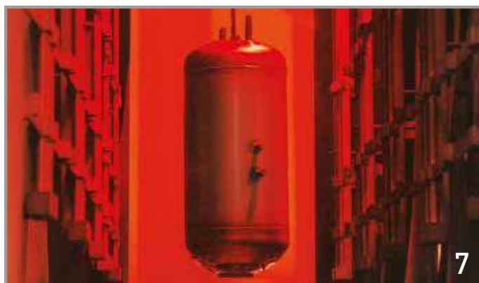
7. Φούρνος ψήσιματος μπόιλερ στους 860°C / Oven boilers heated at 860°C
