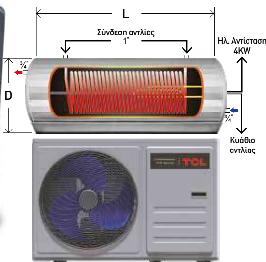
Εξωτερικό κάλυμα αλουμινίου Aluminum exterior cover
